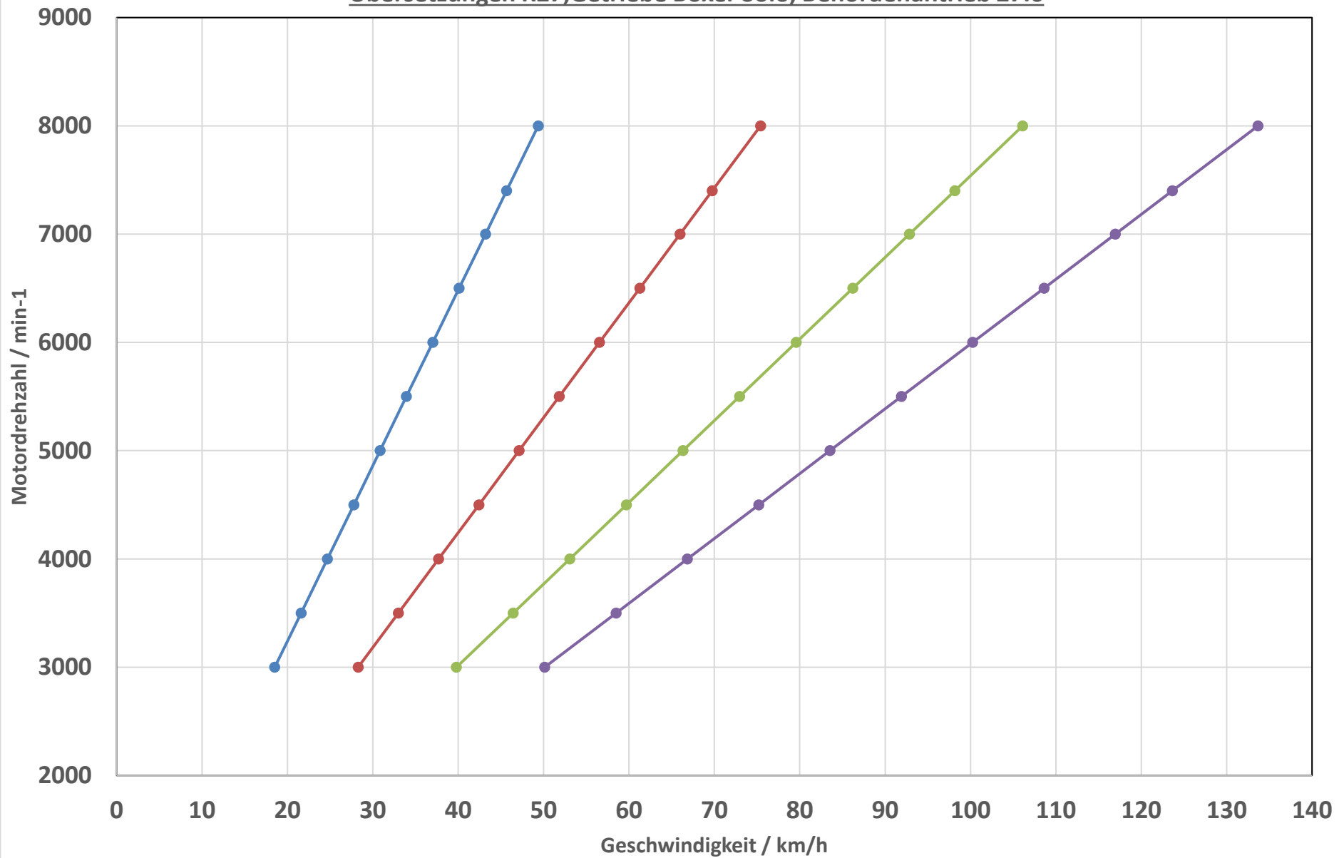
Übersetzungen R27,Getriebe Boxer Solo, Behördenantrieb 27:6
