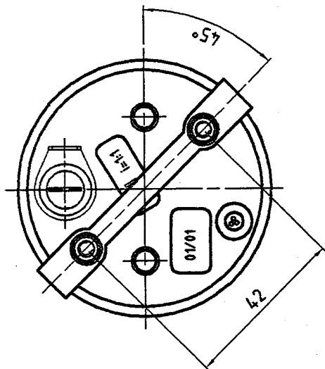
Ansicht mit Einbaubügel
